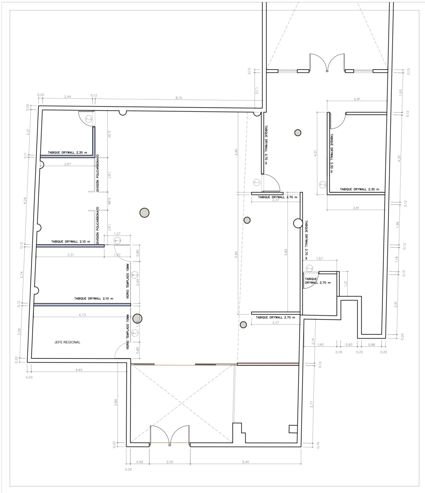
Plano de tabiquería drywall
